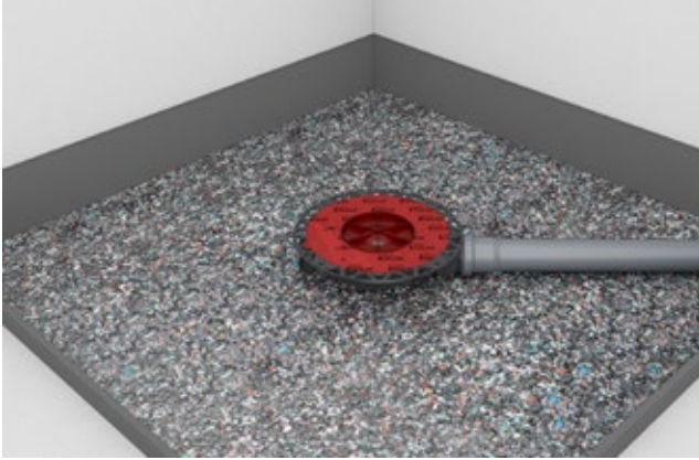
Schritt 1: Vor Einsetzen und Anschluss des Abfalls wird der Untergrund durch Schallschutzmaßnahmen fachgerecht vorbereitet.
