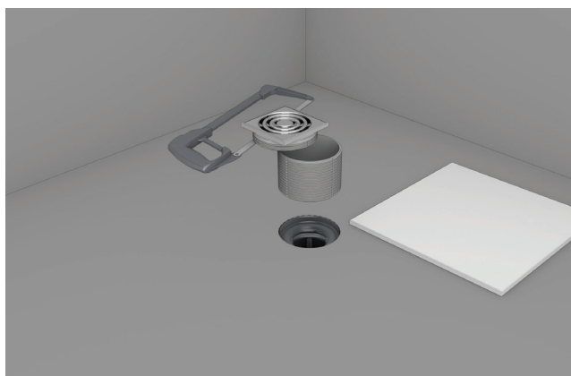
Pasul 5: După ce hidroizolația a fost aplicată complet, înălțătorul pentru sifon este reglat la înălțimea pardoselii.
