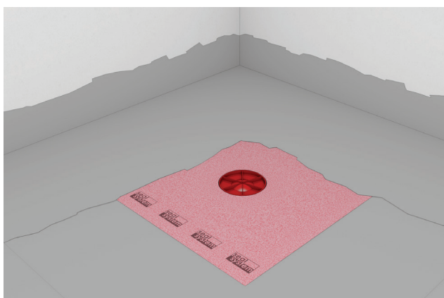
Pasul 4: Membrana de etanșare Seal System este introdusă în primul strat al hidroizolației compozite cât timp acesta este încă umed și apoi se adaugă un nou strat.
