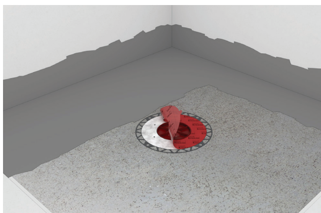
Pasul 3: Folia de protecție este îndepărtată de pe sifon pentru a aplica primul strat de hidroizolație compozită.
