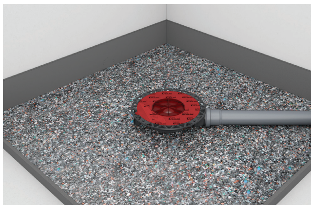
Pasul 1: Înainte de introducerea și conectarea sifonului, baza este pregătită în mod special prin aplicarea covorului de izolare fonică.
