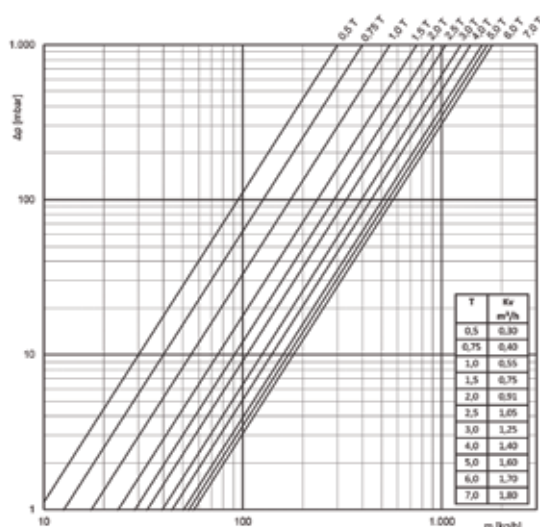
Вентиль на обратную подводу прямой, R 1/2" x Rp 1/2"
